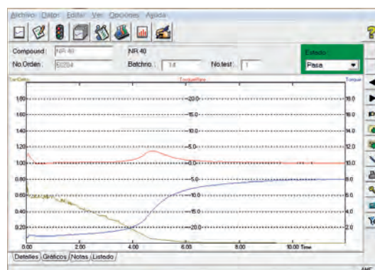
Rheometer
