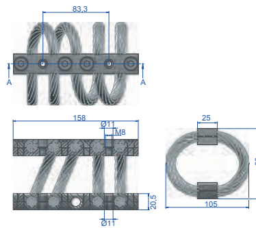
TYPE 158x89
