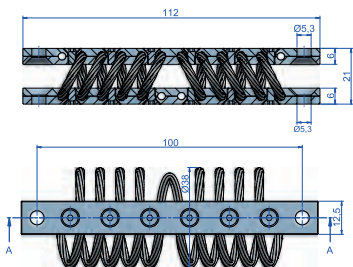
TYPE 112x21
