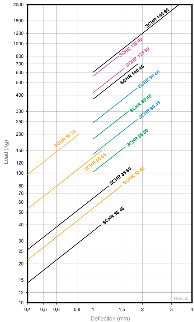
LOAD DEFLECTION GRAPH AMC MECANOCAUCHO® SCHR
